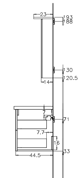
MIRROR CABINET veidrocinē spintelē | peegelkapp | spoguļskapītis
